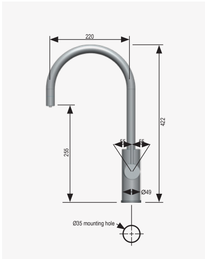
CELSIUS ARC
