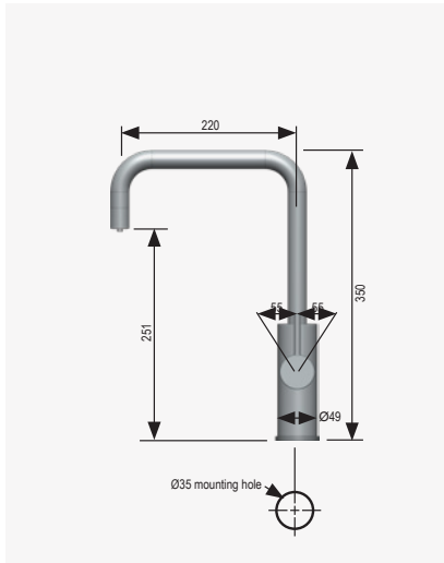
CELSIUS CUBE
